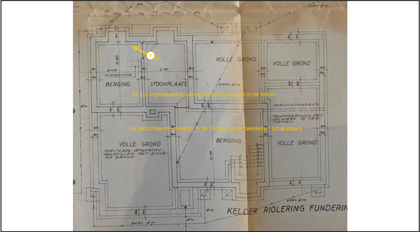
Legende van plan 1.3: Plan kelder
